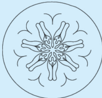
Moon
