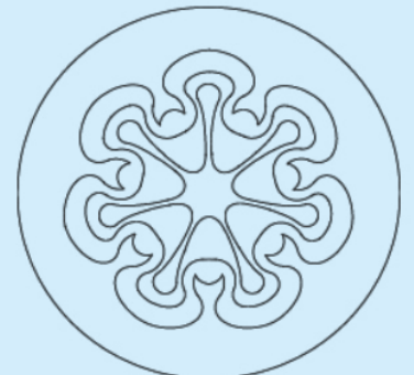
Jupiter
