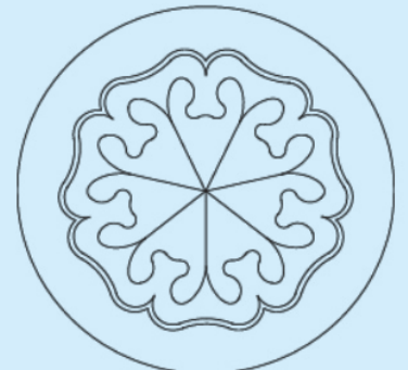
Venus
